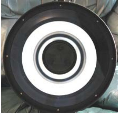
Figure 1. Aspect du miroir avec une bonne collimation.
